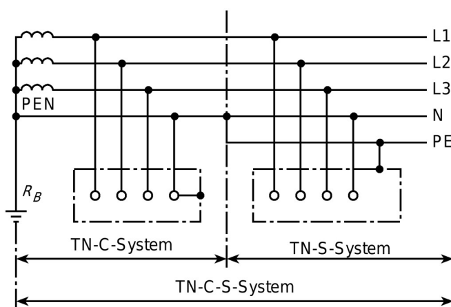
Abb. 13: a) TN-C-S-System
